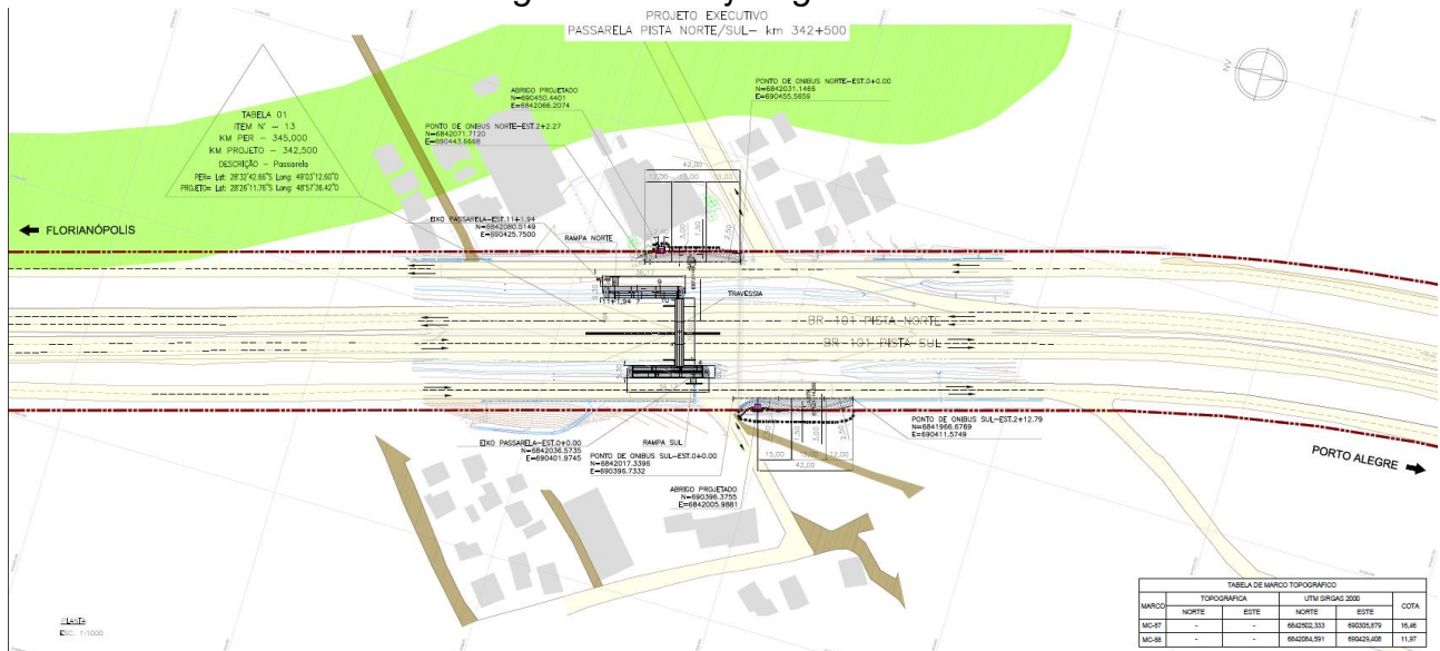
Figura 01 – Projeto geométrico
