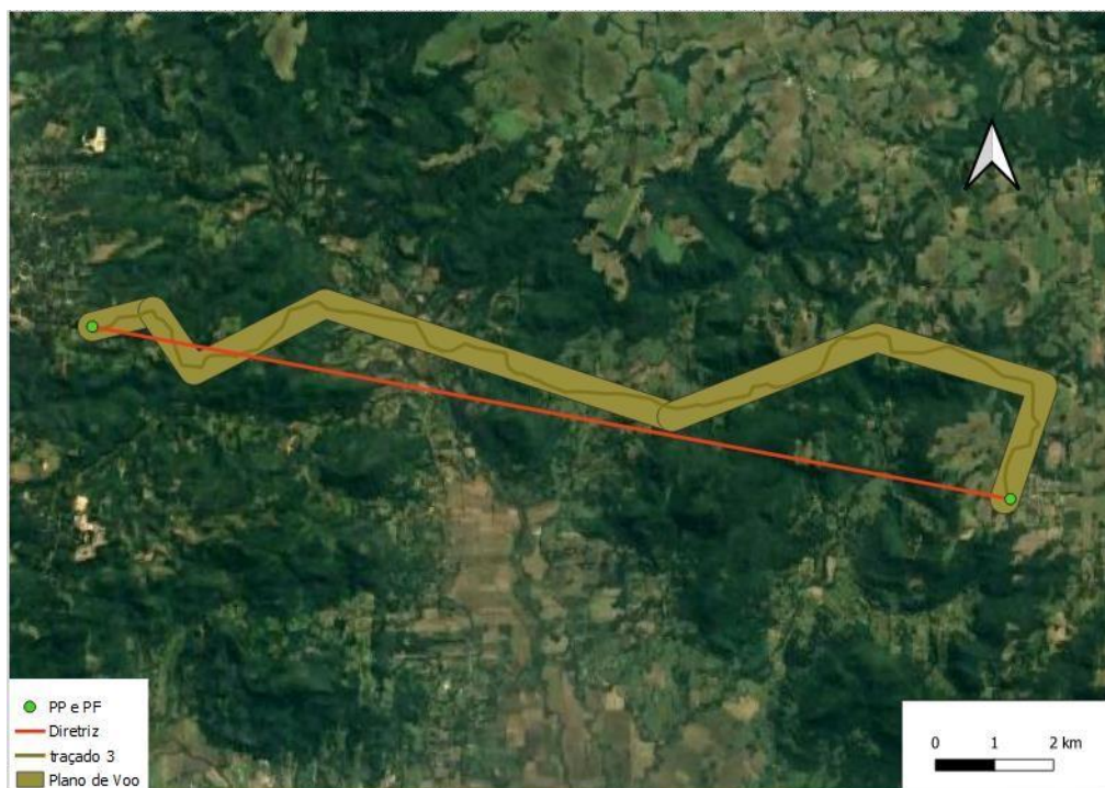
Figura 35: Plano de Voo do Traçado escolhido
