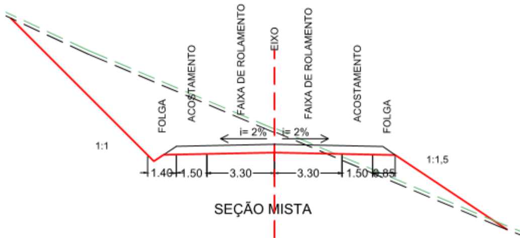
Figura 10: Seção mista
