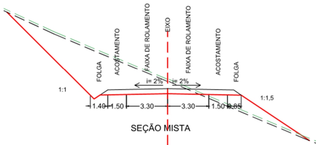
Figura 10: Seção mista
