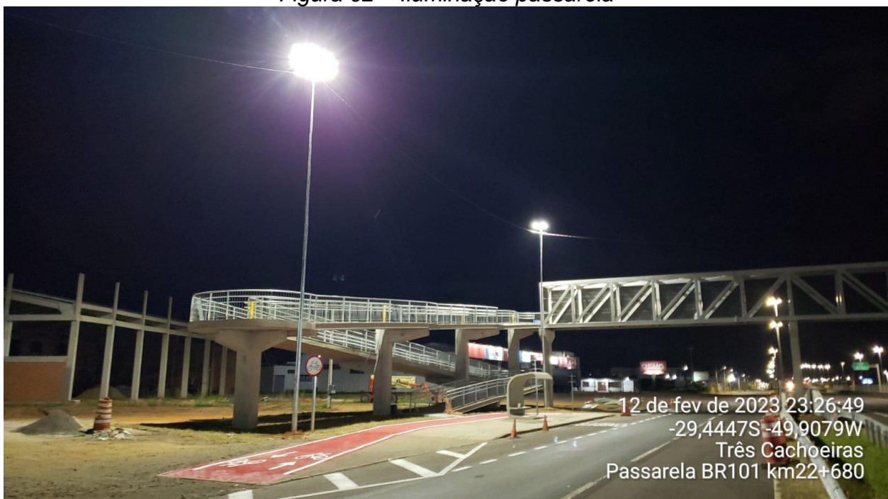
Figura 02 – Iluminação passarela
